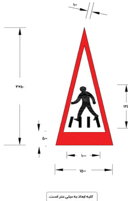
شکل ۵-۱-۹- جزئیات نماد اخطاری خطر عبور عابرین پیاده به تفکیک انواع راه‌ها
