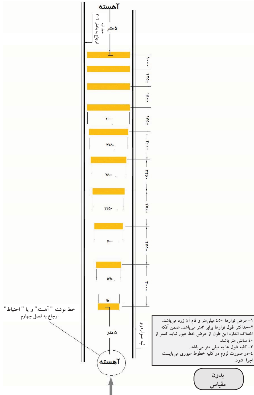
شکل ۳-۶-۱- جزئیات خط کشی نوارهای عرضی میله‌های در خط عبور
