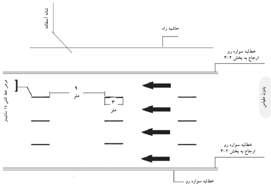
شکل ۲-۲-۲- خط کشی خط عبور در معابر بزرگراهی و آزادراهی
