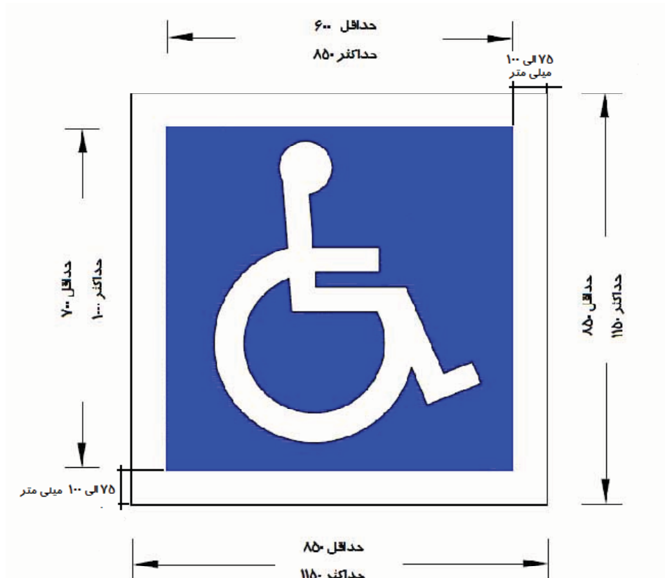
شکل ۵-۱-۱- جزئیات مربوط به نماد ترافیکی ویژه معلولین
