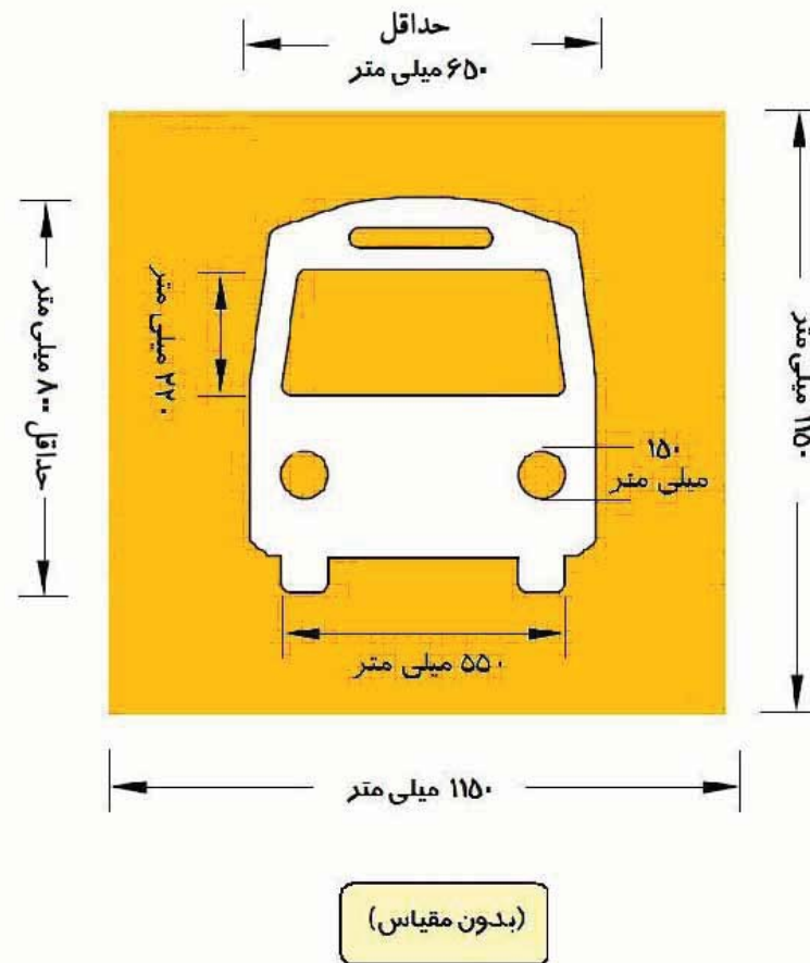
شکل ۵-۱-۸ - جزئیات خط کشی نماد خط ویژه اتوبوس
