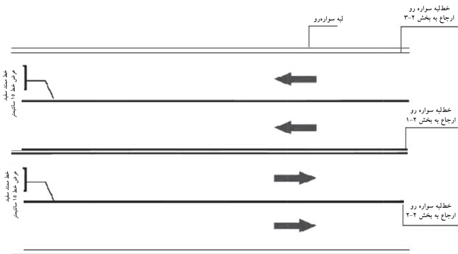
شکل ۲-۲-۲- خط کشی خط عبور در معابر بزرگراهی و آزادراهی
