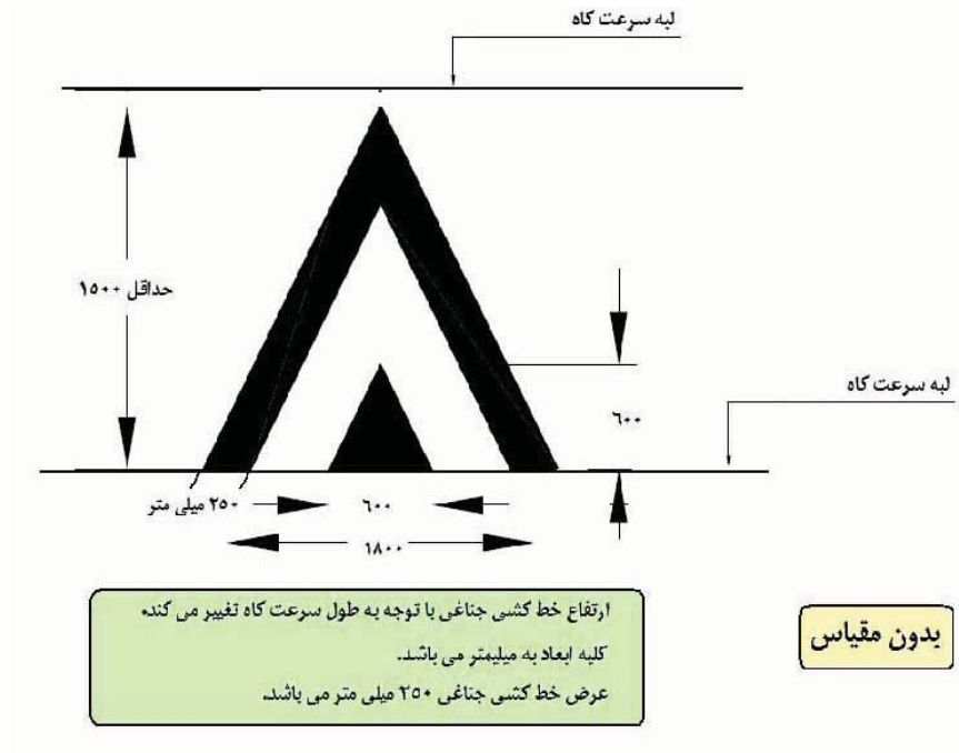
شکل ۳-۵-۱- خط کشی سرعتگاه ، الف) جزئیات نماد
